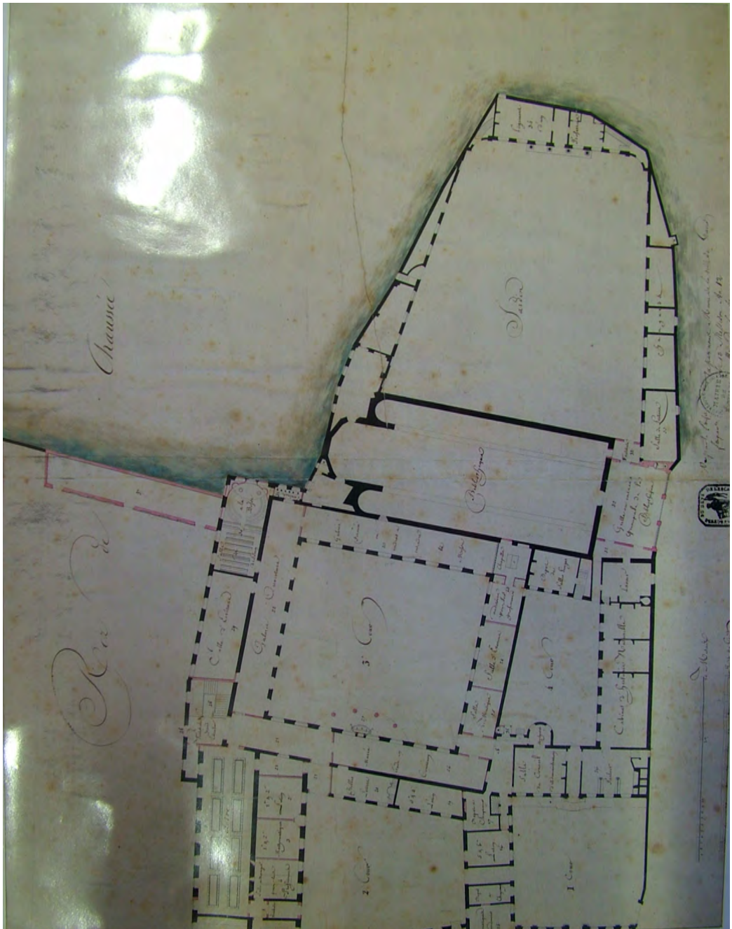
Fig. 5. Plan voor de verbouwingen naar Lycée door Pisson, 1804, het gelijkvloers (SAG, L129/3).
