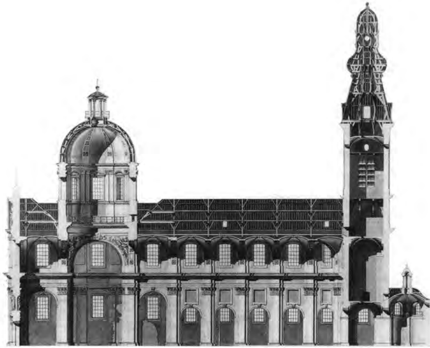
Fig.16. Sint-Pieterskerk, langdoorsnede, begin 20ste eeuw. (SAG)
