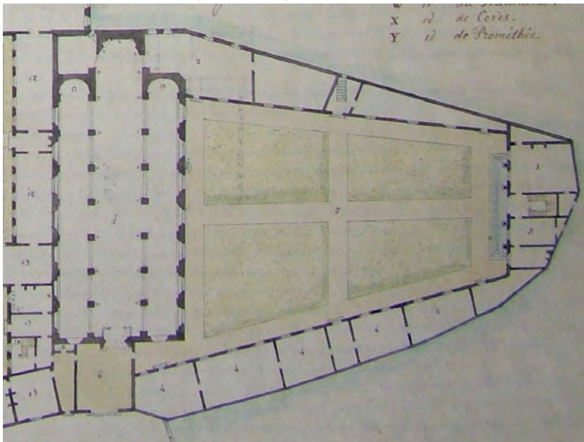
Fig.11. Plan van De Noter, 1818, een detail. Dit sterk vereenvoudigde plan toont de graad van uitvoering van het project van Pisson. De leeszaal in de voormaligesacristie staat rechts van het koor. (SAG, L129/5)
