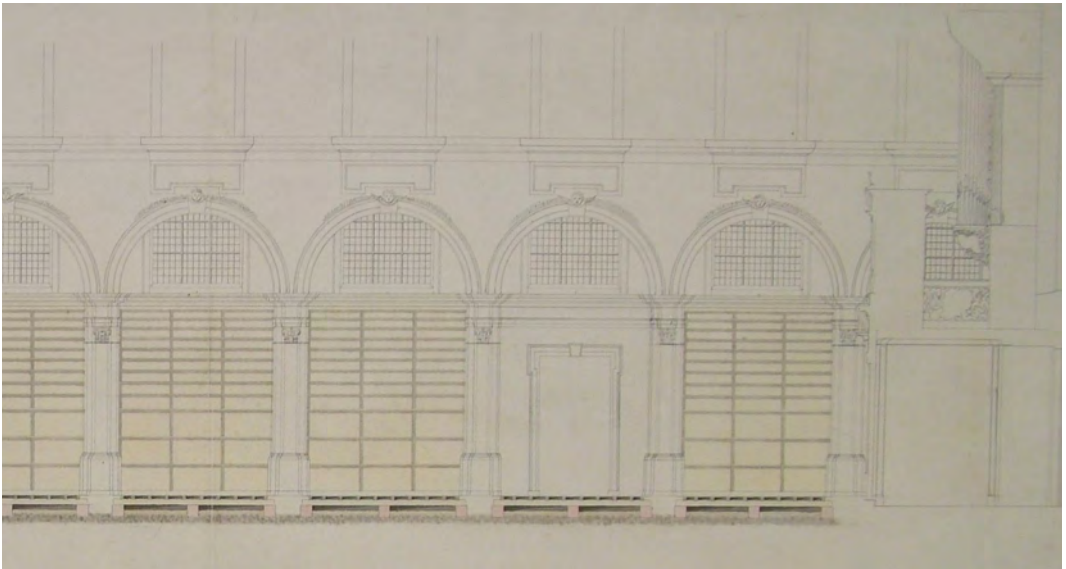
Fig.11. Doorsnede van de hand van Roelandt voor interieurwerken in 1818. De tekening, met rechts het orgel, geeft een goed beeld van hoe de bibliotheek er vanaf 1801 moet hebben uitgezien. (UG, kaartenzaal, map 'bibliotheek van de universiteit')
